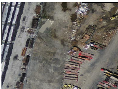
WGS84 経度緯度に変換した後 ( wgs_84 )
