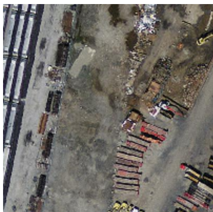
元のラスタはメートル単位のマサチューセッツ州平面 ( mass_stm )
