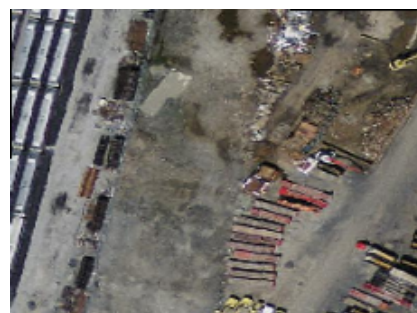
最近傍補間の代わりに双線形補間を使って WGS84 経度緯度に変換した後 ( wgs_84_bilin )
