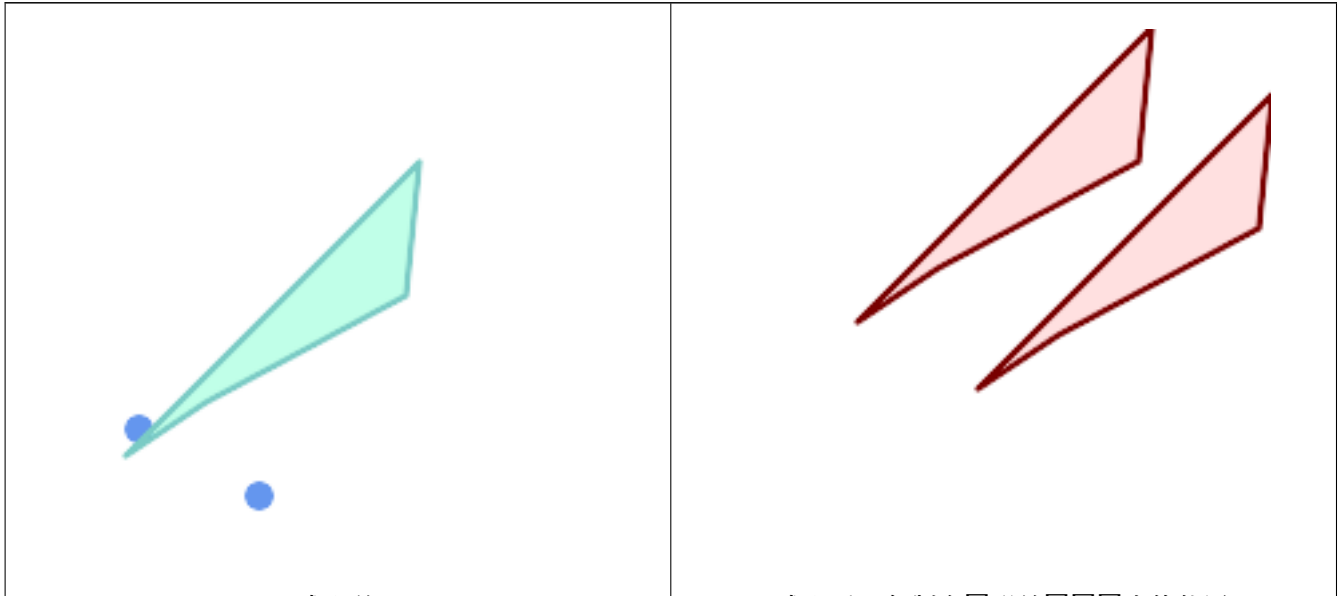
求和前
