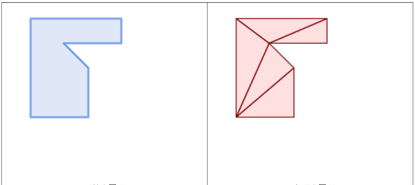
原始多边形
