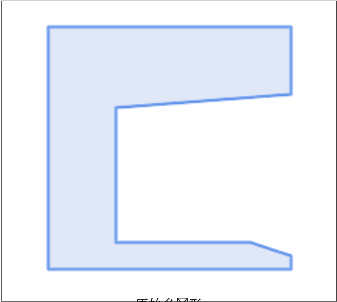
原始多边形
