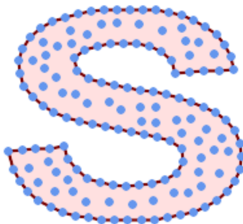
多点的凹壳
