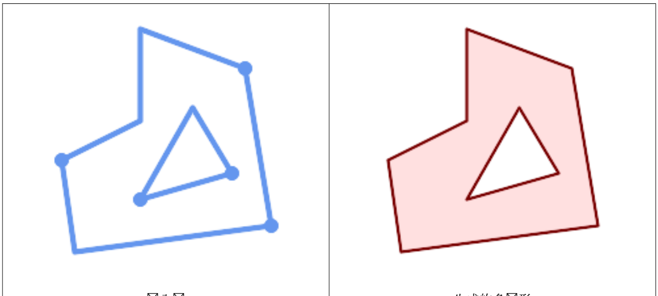
输入
