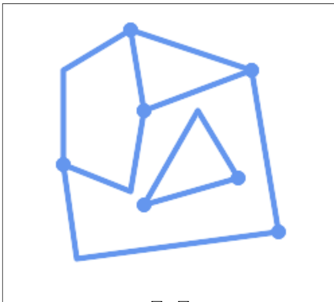
输入
