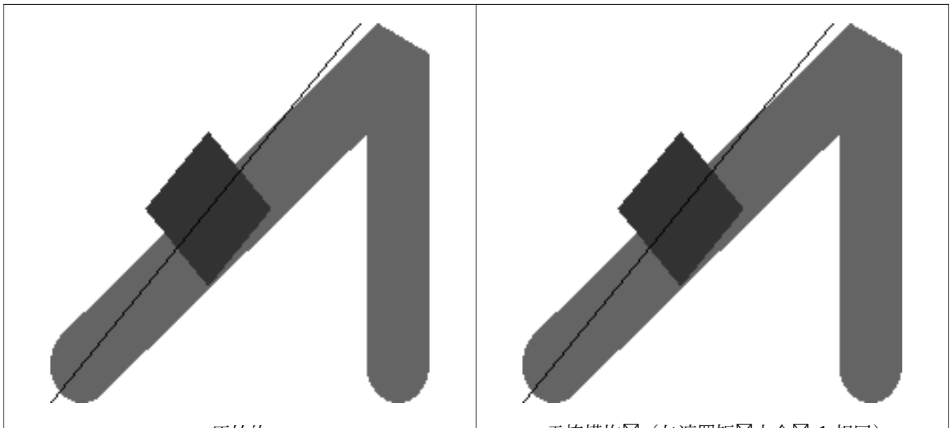
原始的
