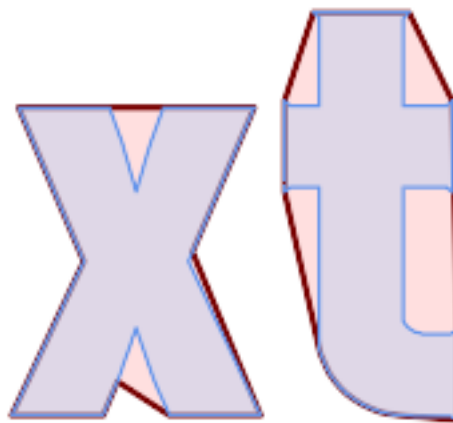
Simplification de l'enveloppe extérieure d'un MultiPolygone, avec segmentation
