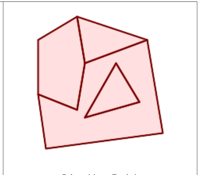
Polygonisiertes Ergebnis
