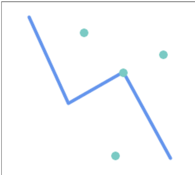
MEHRPUNKT / LINESTRING
