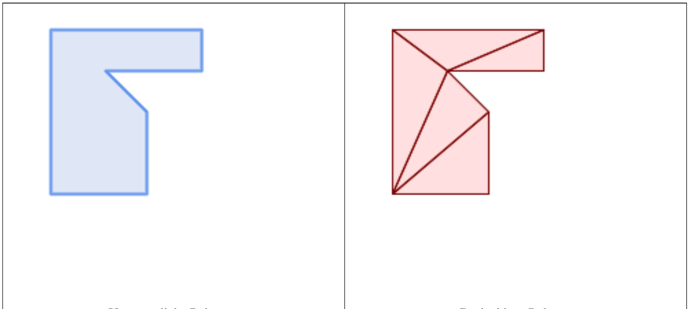
Ursprüngliche Polygone
