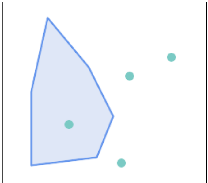
MEHRPUNKT / POLYGON
